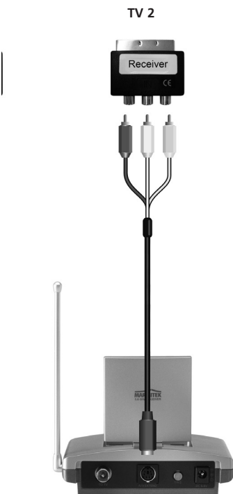
Afbeelding 2 A/V ONTVANGER
