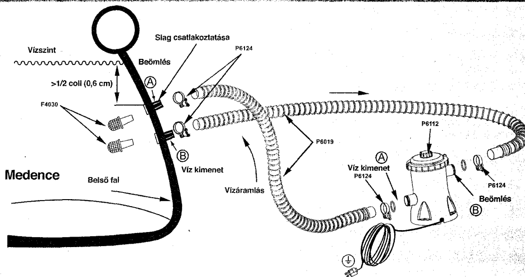
A medence és a szűrőkosaras szivattyú ábrája (nem arányos)
