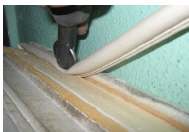
szilikongumi tömítés behengerlése
